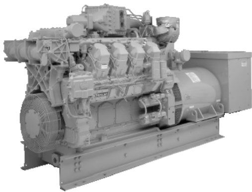
Генераторная установка показана с оборудованием, устанавливаемым по специальному заказу
